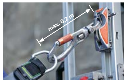
15 Läufer eines Steigschutzsystems.
