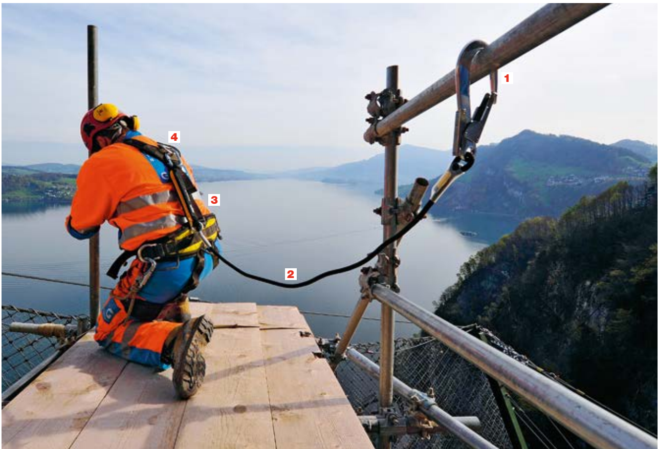
1 Absturzsicherung.
