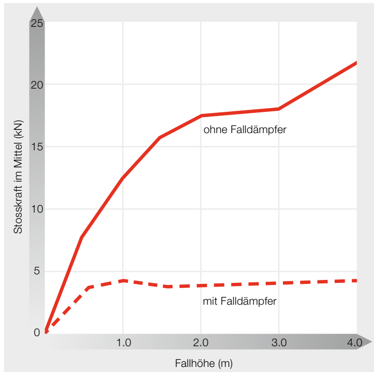
2 Fangstoss bei Fallversuchen, in Abhängigkeit von der Fallhöhe.
