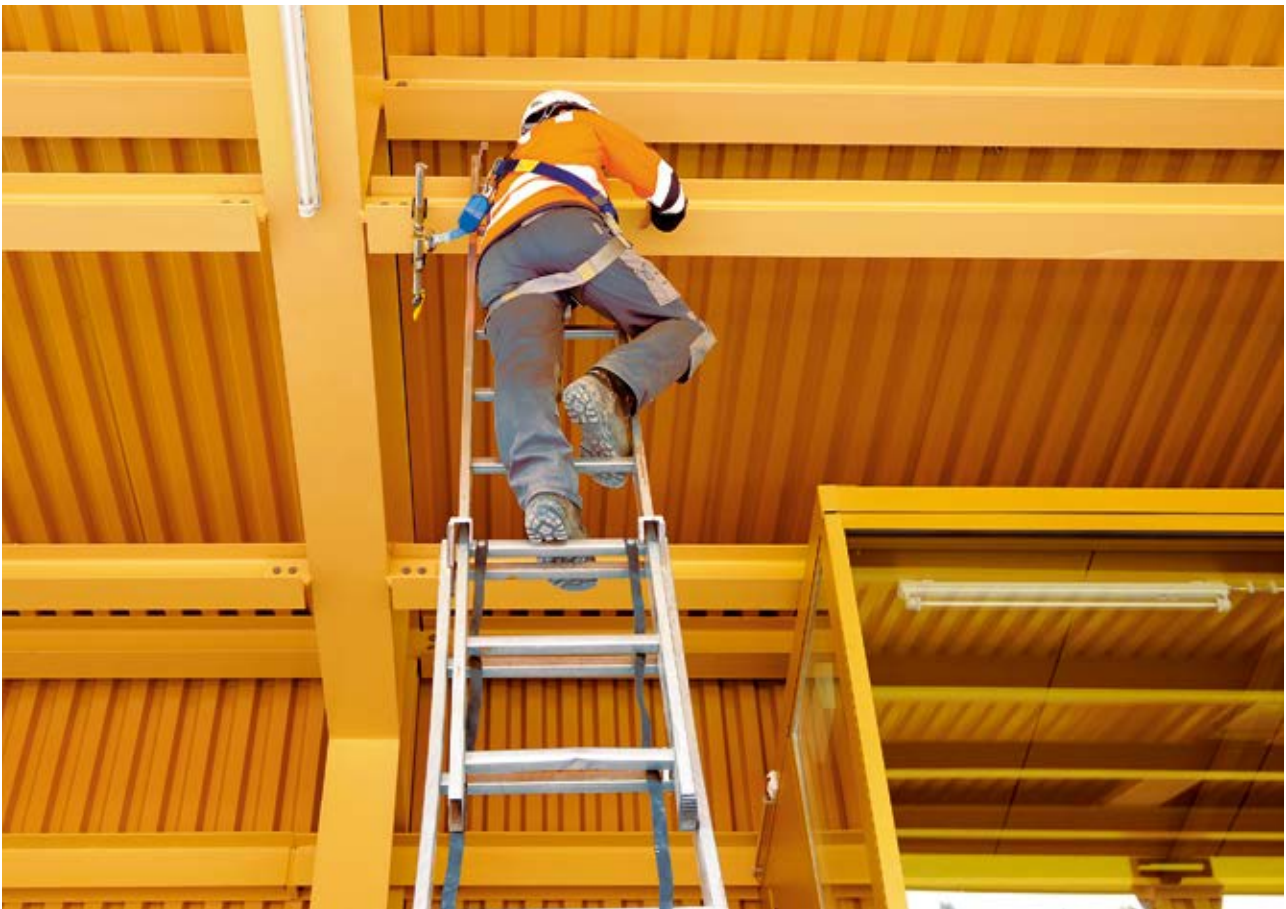
27 Gesichertes Arbeiten auf einer Leiter mit Höhensicherungsgerät und mobilem Anschlagpunkt.
